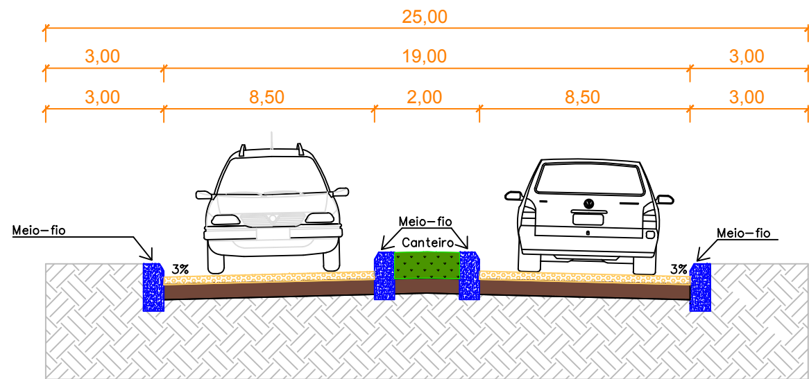
SEÇÃO TRANSVERSAL AVENIDA INOCÊNCIO PEREIRA DE BRUM SEM ESCALA
